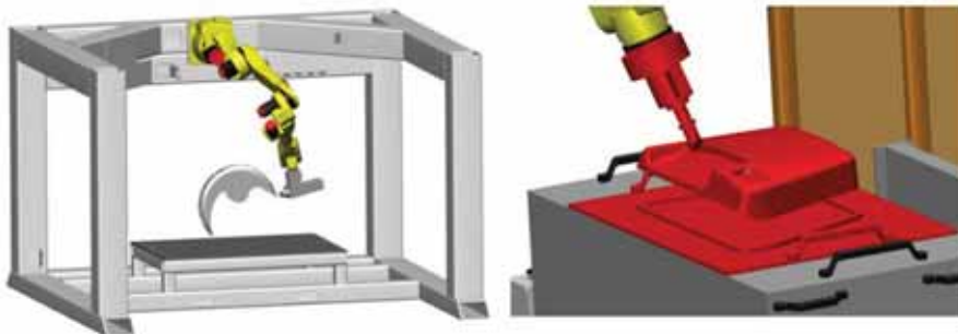
RobotMaster'la Robot üzerinde gerçek zamanlı işleme simülasyonu
