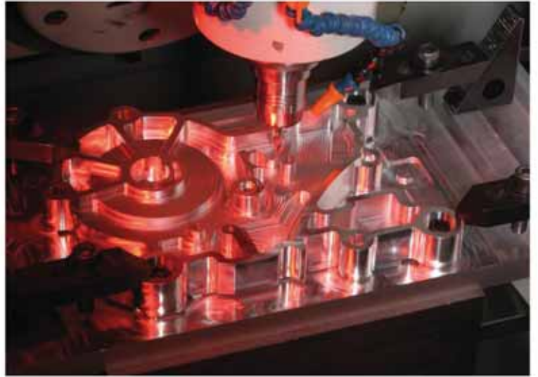
Mastercam for SolidWorks'te İşlenmiş Parça
